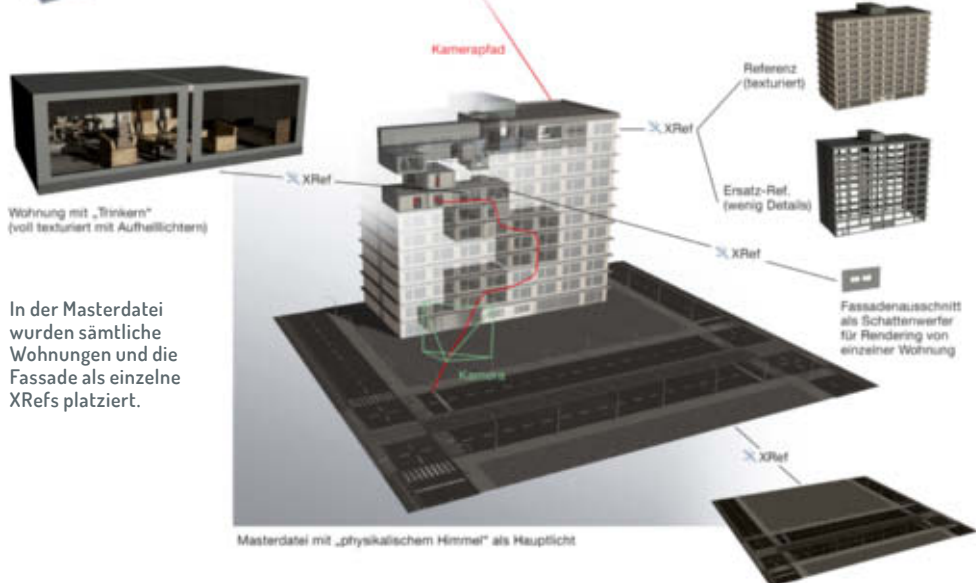
Das gesamte Gebäude wurde mit allen wichtigen Details als „Rohbau“ angelegt.
